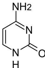
Cytosine
