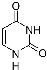
Uracile
